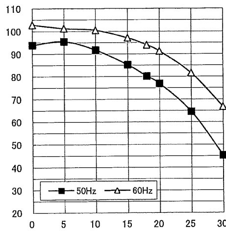
圧力～入力特性
