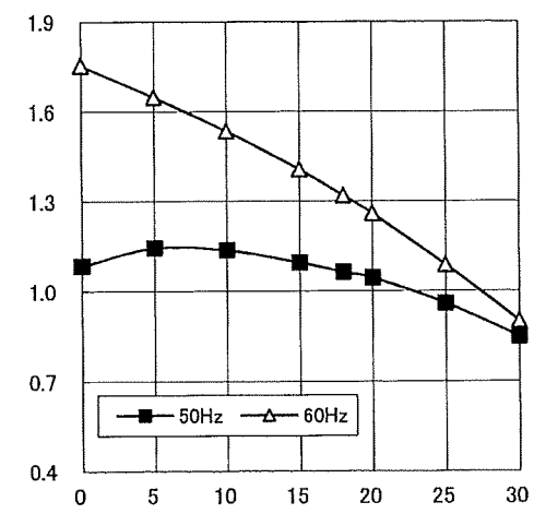
圧力～電流特性
