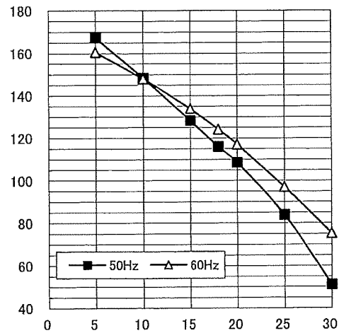
圧力～風量特性
